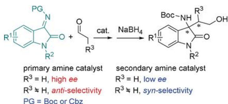
图 2、高对映选择性的 Mannich 反应
