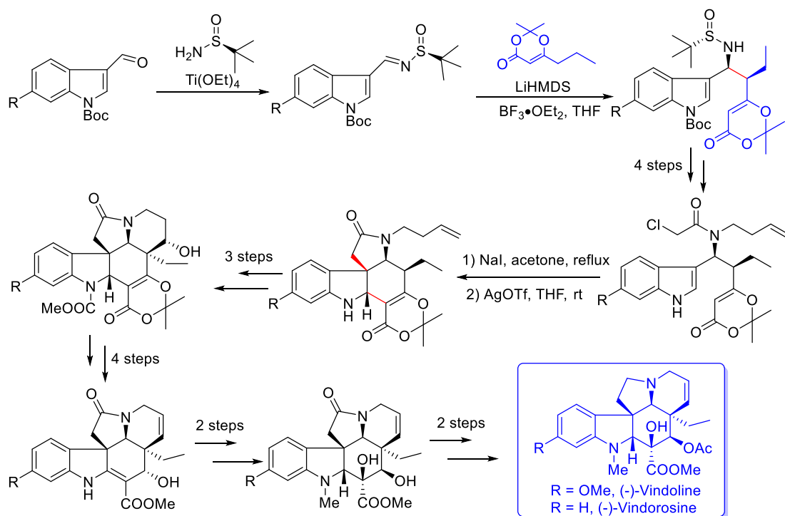
图 1、Vindoline 及 Vindorosine 的全合成
