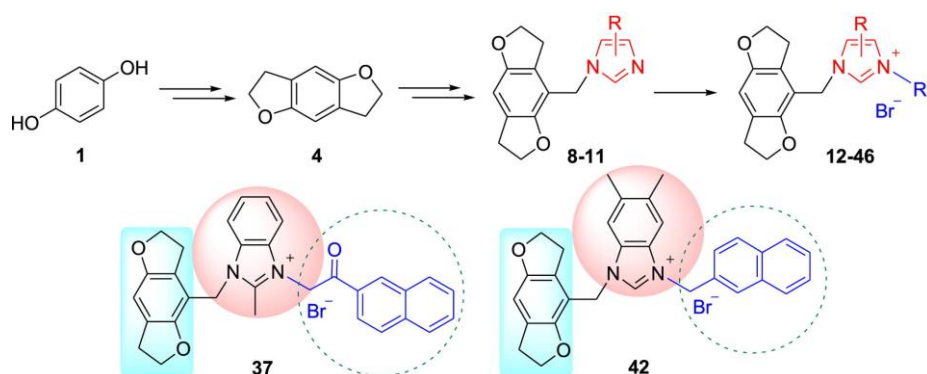
图 4、四氢苯并二咪唑—咪唑盐的合成与抗肿瘤活性研究
