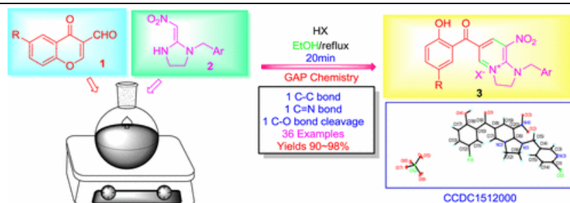
图 3、基于氮杂烯酮的杂环绿色环保的合成方法
