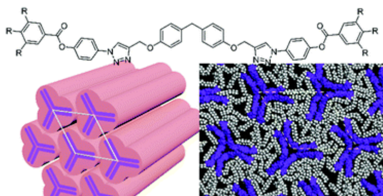
图 7、弓形多链型化合物形成具有非中心对称 p31m 结构的柱相液晶
