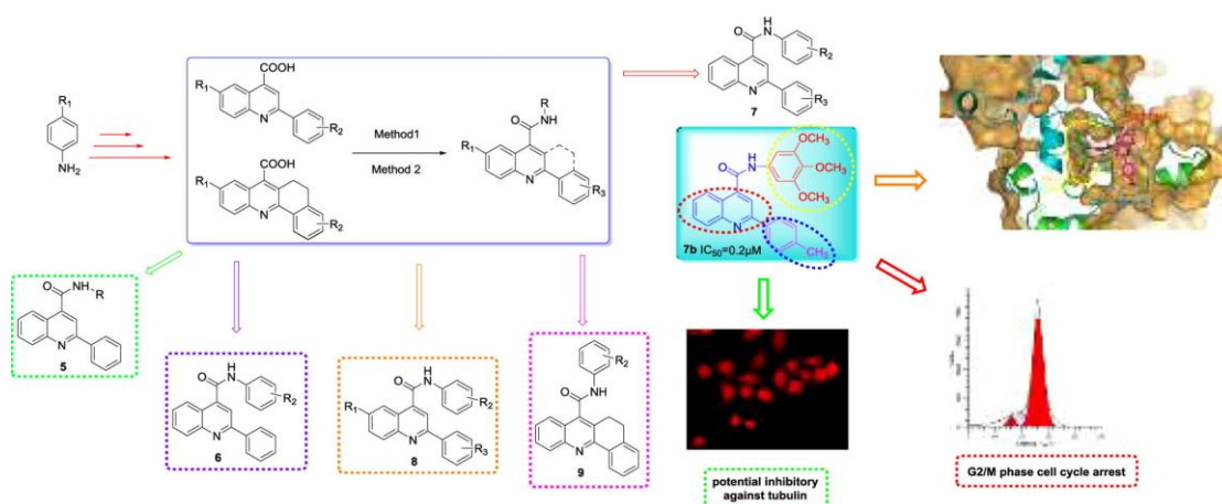
图 5、新型苯基喹啉类衍生物的合成、抗肿瘤活性与作用机制研究
